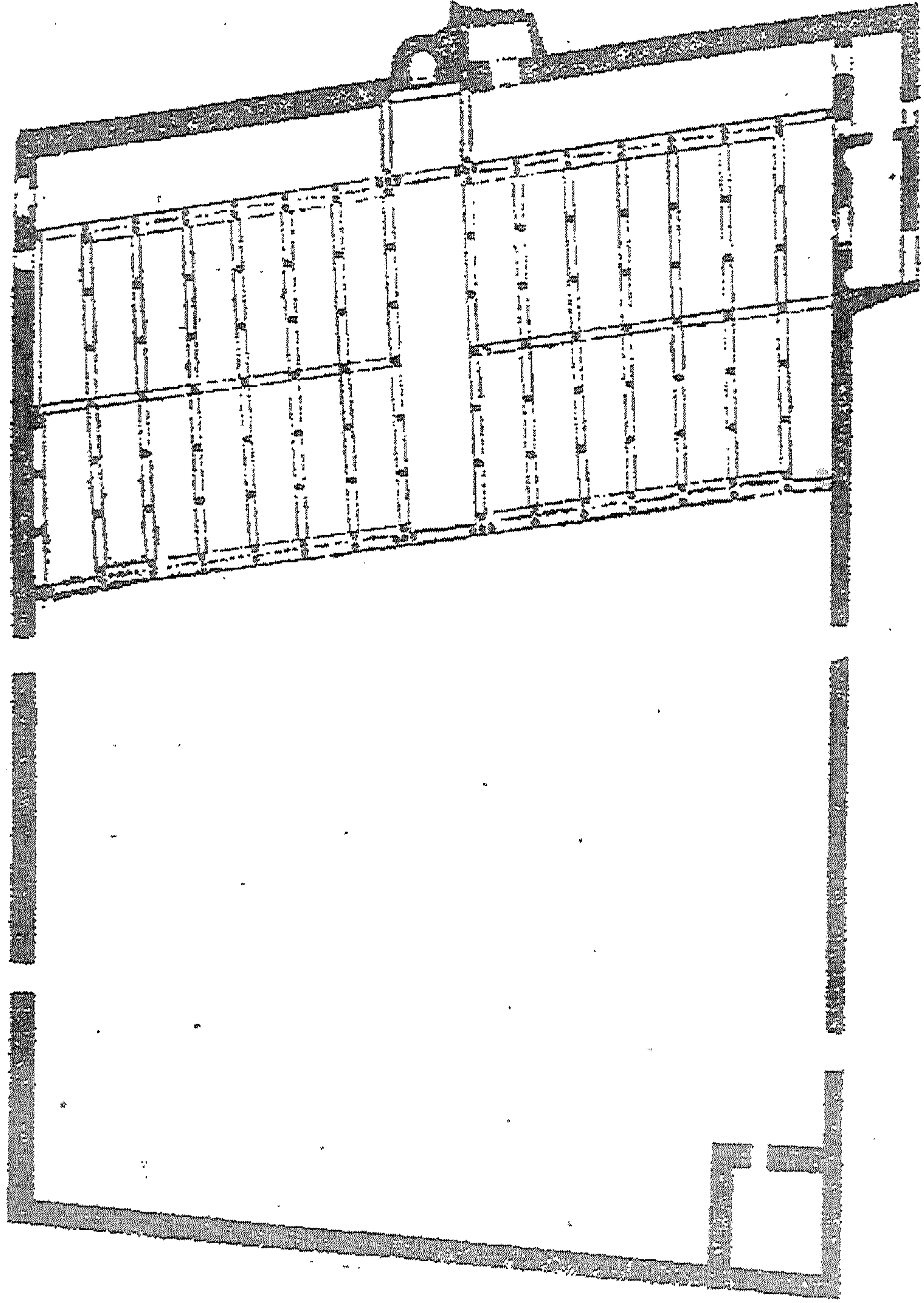
(شكل رقم ٦٠) رسم تخطيطي لجامع الزيتونة في عهد الأغالبة عن د/احمد فكري
